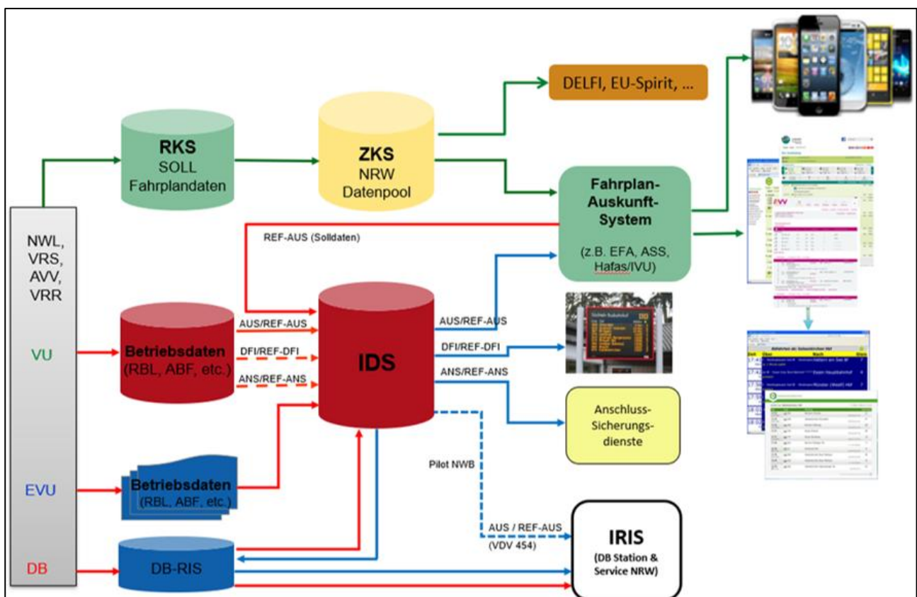
Abbildung 5: Schematische Darstellung eines Fahrplanauskunftssystems am Beispiel des VRR
