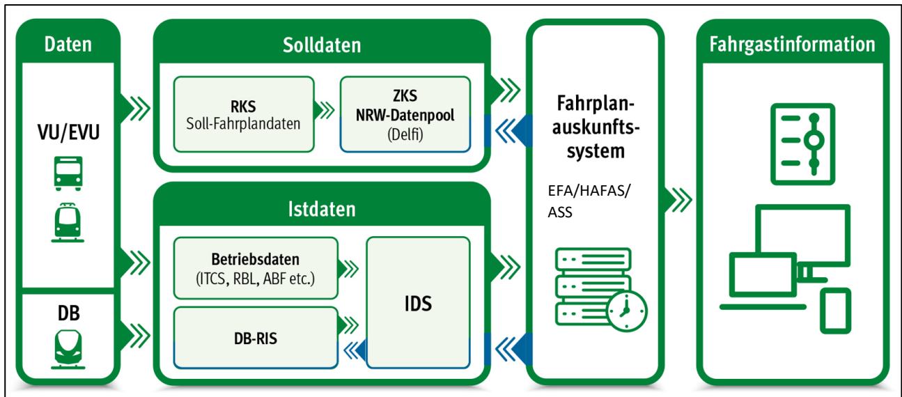
Abbildung 6: Schematischer Datenfluss IST- und Solldaten
